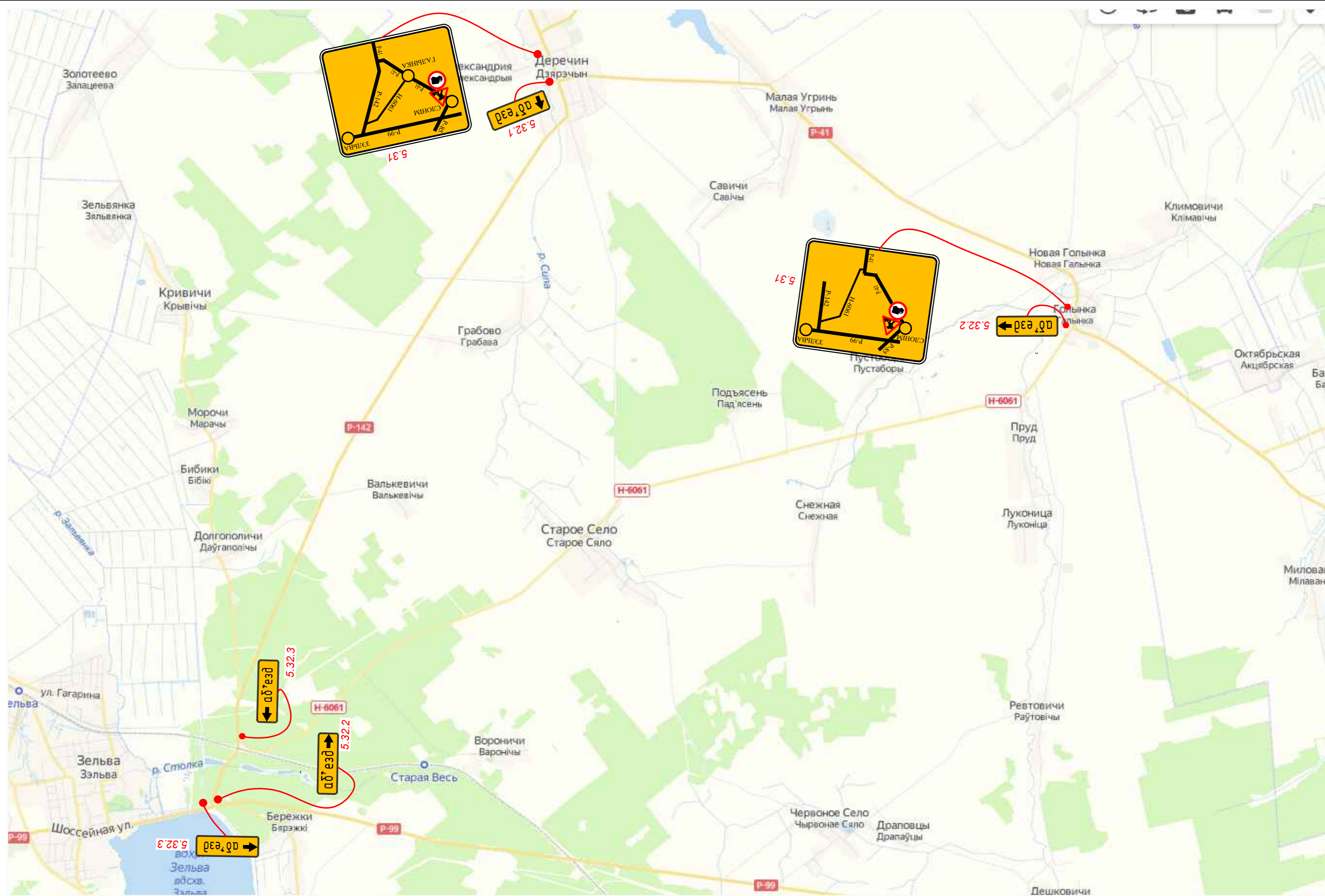
1. Схема организации дорожного движения на время проведения работ выполнена согласно ТКП 636-2019
